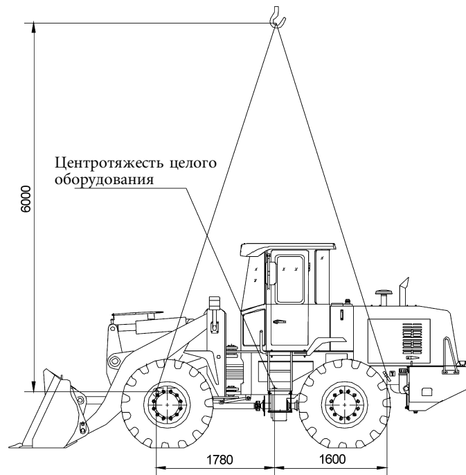
Рис.3-4 Схема подъема целой машины
